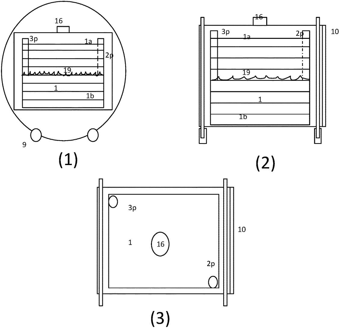
FIG 8A RA=0
